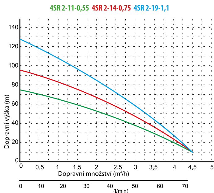
Výkonostní tabulka čerpadel 4SRm / 4SR
